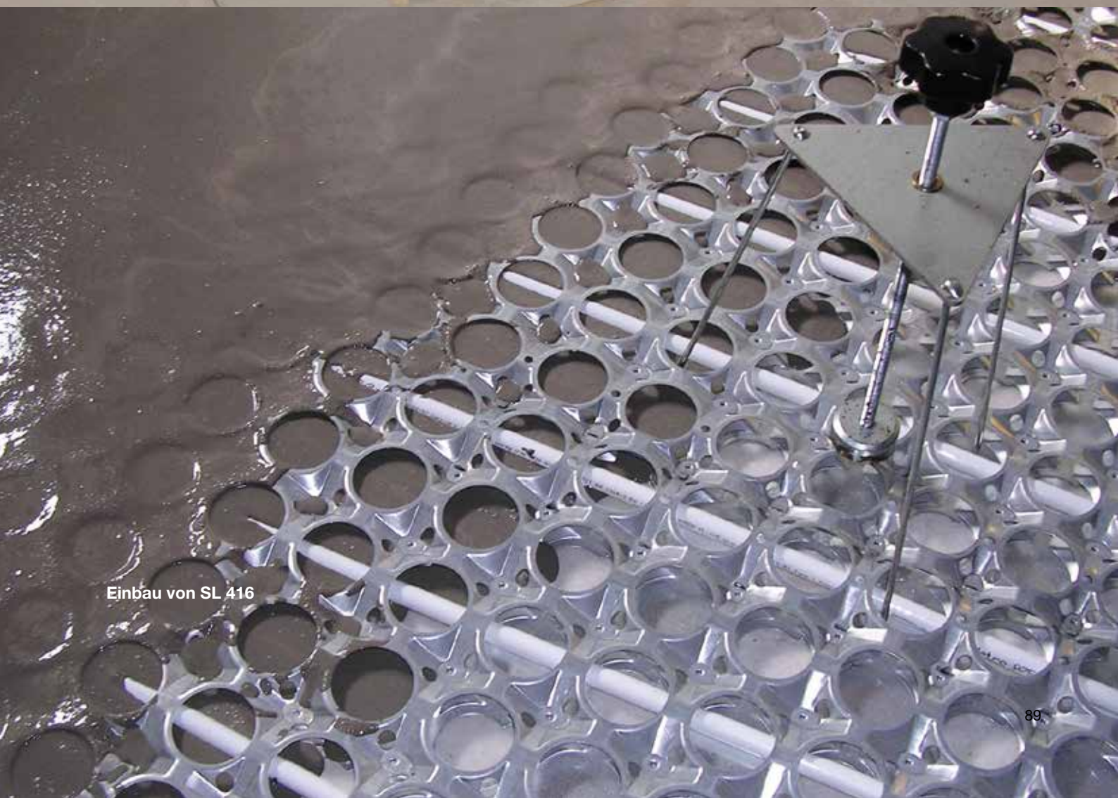
Einbau von SM 485 auf einer Fußbodenheizung
