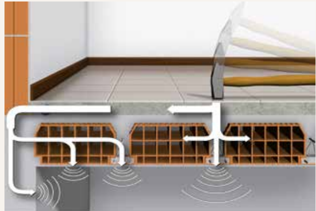
Ausbreitung des Schalls über die Struktur eines Gebäudes mit einschichtigem Estrich
